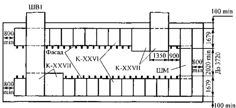
Рис. 6.3.19. Вариант двухрядного размещения камер серии К-XXVII с камерами серии К-XXVI: ШВІ — шинные вводы на секцию шин; ШМ — шинный мост между двумя рядами камер
