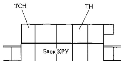
Рис. 6.5.10. Вариант установки отдельно стоящих шкафов трансформаторов собственных нужд и трансформаторов напряжения
