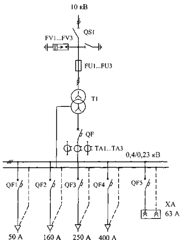
Рис. 4.3.31. Однолинейная электрическая принципиальная схема КТПК (ВК)-400/10/0,4-91-У1 производства Самарского завода «Электроштит»: FU1—FU3 — предохранитель; FV1—FV3 — разрядник; QF — автоматический выключатель; QS1 — разъединитель; QF1—QF5 — автоматический выключатель; TI — силовой трансформатор; TA1—TA3 — трансформатор тока
