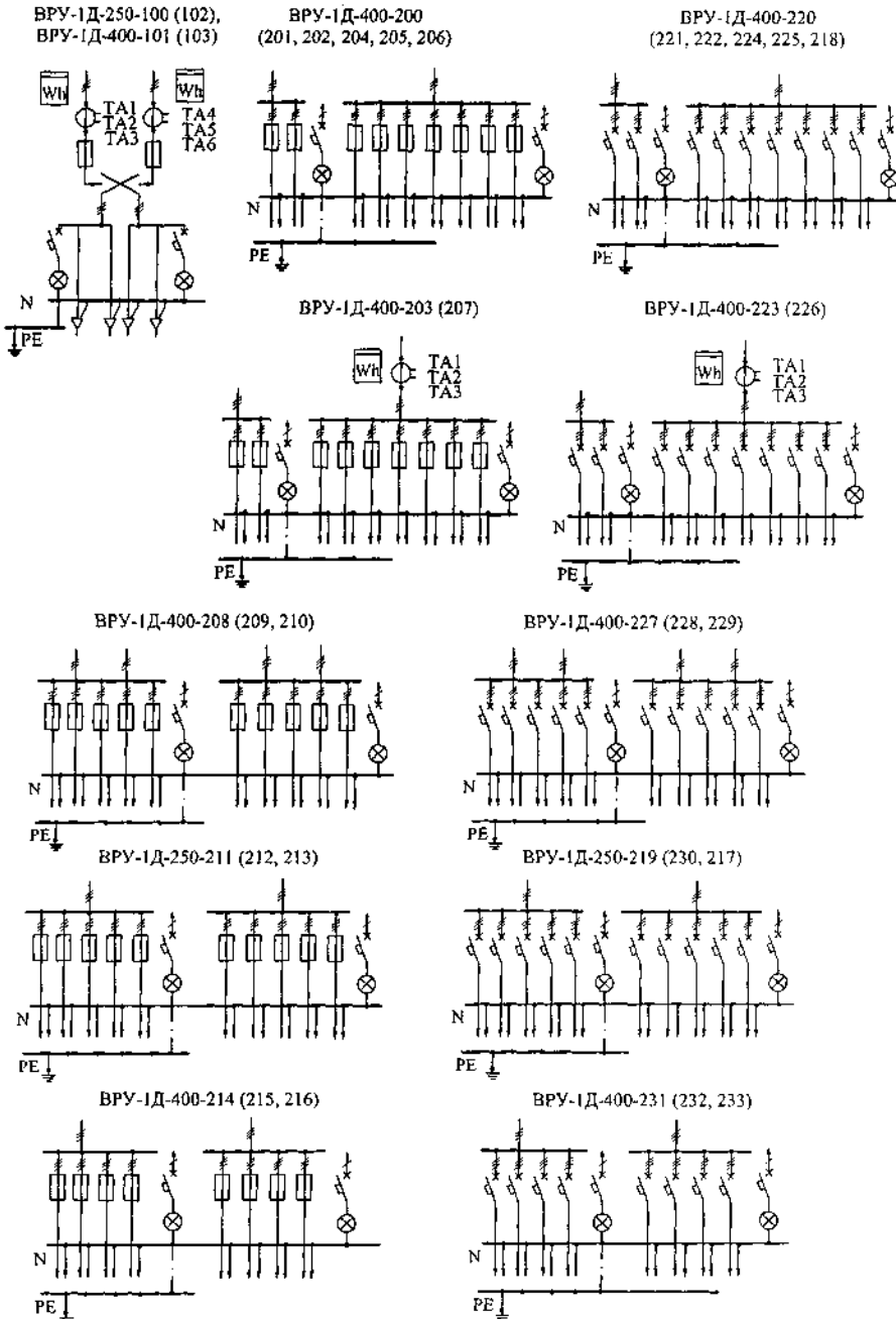
Рис. 7.4.2. Принципиальные схемы вводно-распределительных устройств серии ВРУ-1Д производства Дивногорского завода низковольтной аппаратуры (Начало, продолжение см. стр. 371, 372)
