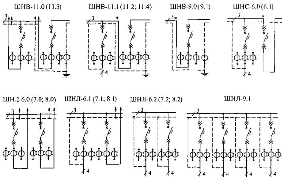
Рис. 4.3.11. Схемы соединений шкафов РУНН КТПП 1600 кВ·А производства Самарского завода «Электроцит»
