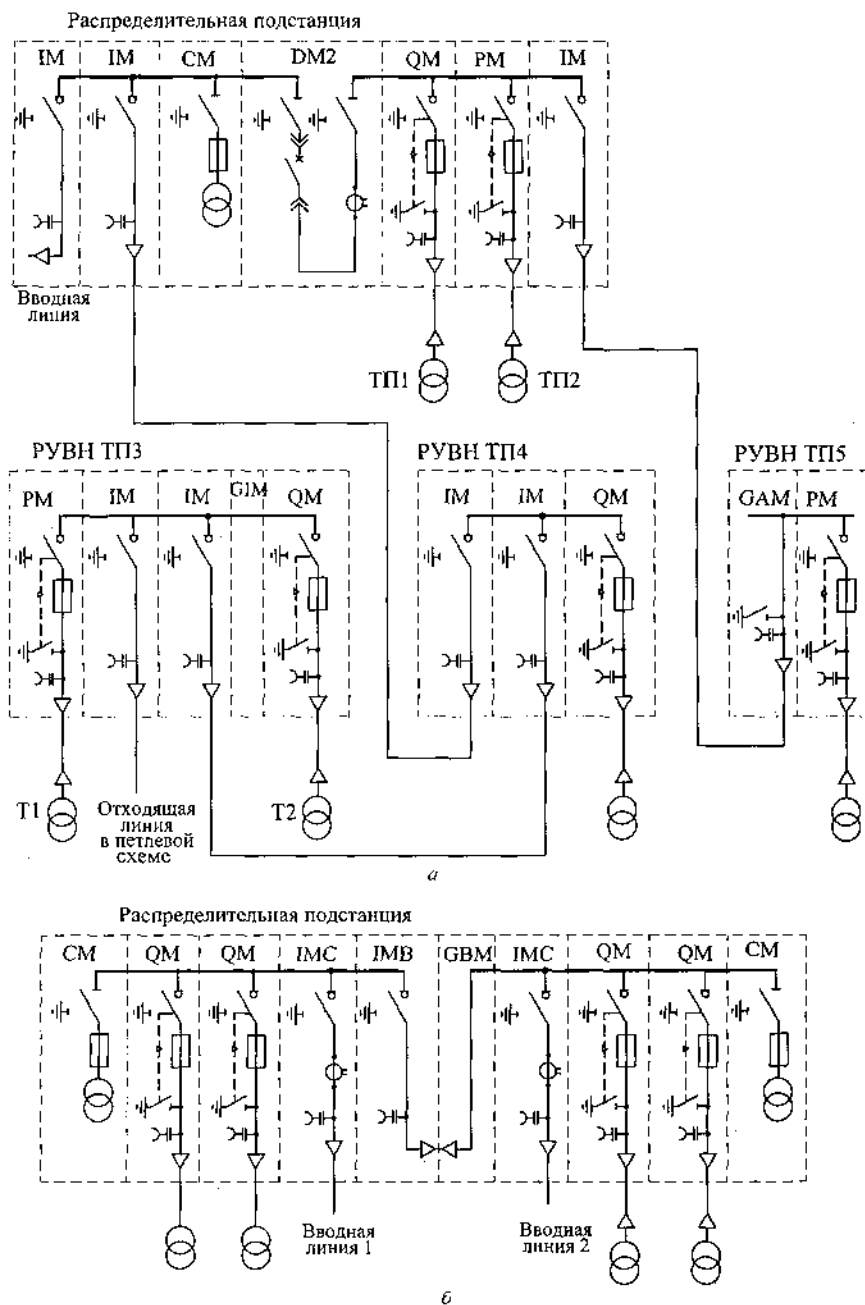
Рис. 6.6.12. Примеры принципиальных схем РП и РУВН трансформаторных подстанций: a — распределительной сети; б — распределительной подстанции
