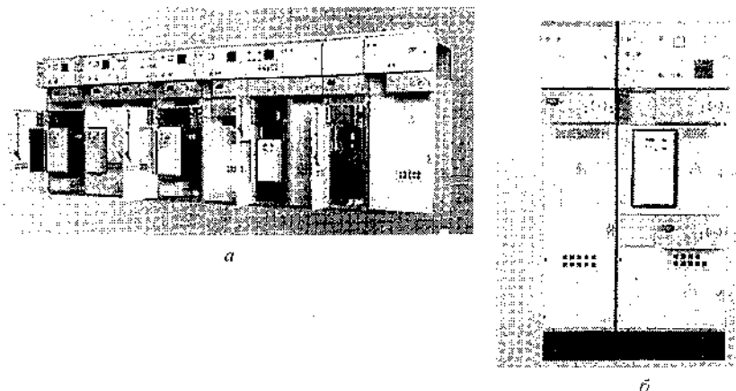
Рис. 6.2.6. Общий вид распределительного устройства (а) и камера КСО-6(10)-Э1 «Аврора» (б)
