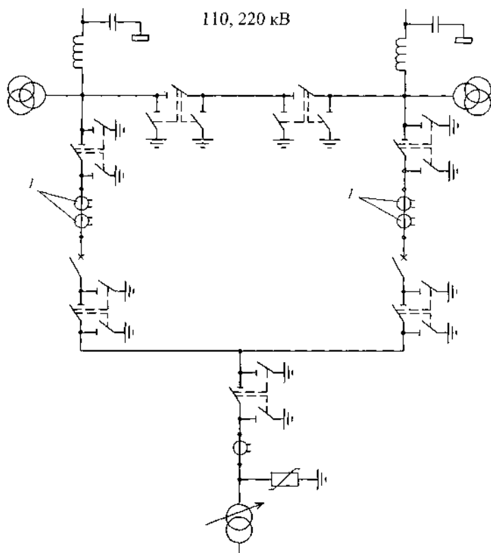
Рис. 3.4.16. Схема «заход—выход»: T — трансформаторы тока, установка которых должна быть обоснована (индекс схемы — 6 по [26])
