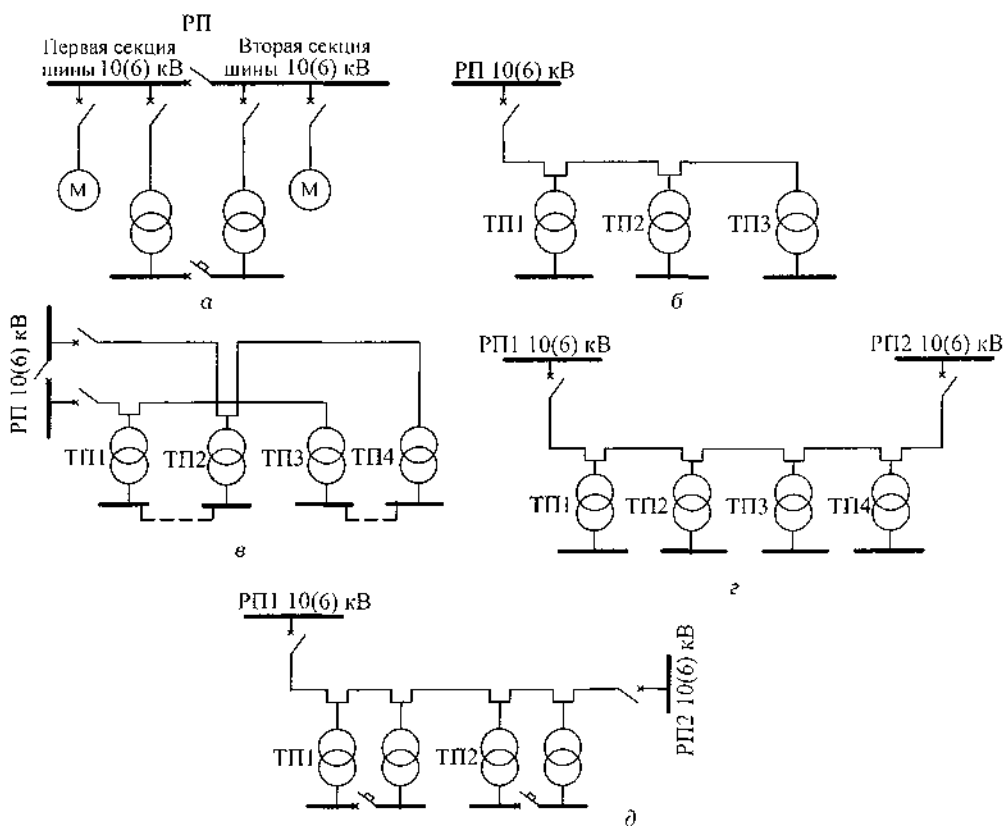
Рис. 1.8.2. Схемы питания ТП 10(6) кВ: а — радиальная; б — односторонняя магистраль с односторонним питанием; в — односторонняя магистраль с частичным резервированием по связям вторичного напряжения; г — петлевая для питания однотрансформаторных ТП; д — для питания двухтрансформаторных ТП
