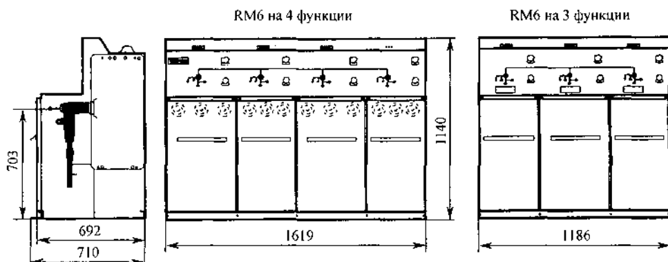
Рис. 6.6.17. Размеры моноблока RM6 без возможности расширения
