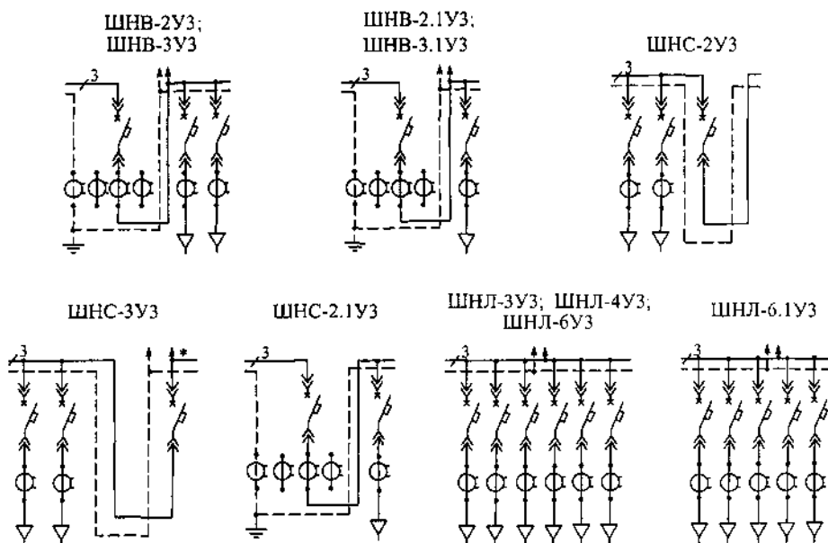
Рис. 4.3.10. Схемы соединений шкафов РУНН КТПП 250—1000 кВ·А производства Самарского завода «Электроцит» (шкафы для КТПП с изолированной нейтралью выполняются без связи с нейтралью)
