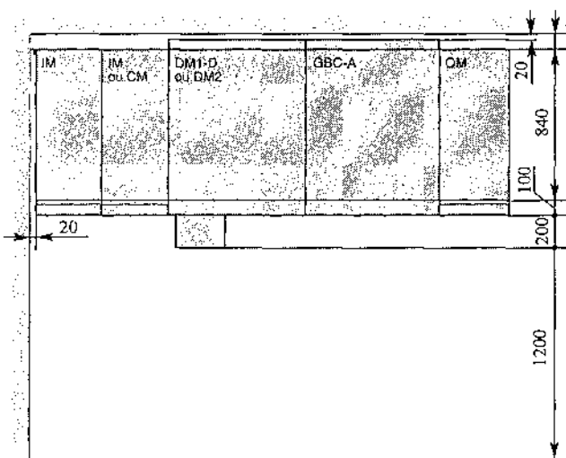
Рис. 6.6.11. Примеры компоновок распределительных устройств с ячейками SM6
