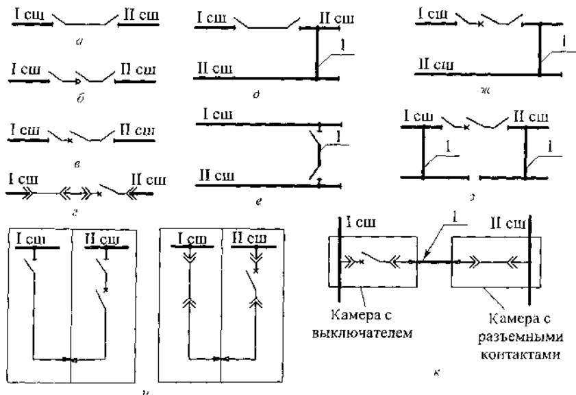
Рис. 6.8.4. Вариант секционирования сборных шин при однорядном ( а–г ) и двухрядном ( д–и ) расположении камер: а, д, е — с разъединителями; б — с разъединителями и выключателем нагрузки; в, ж, з — с разъединителями и высоковольтным выключателем; г — с высоковольтным выключателем выкатного исполнения; и — камеры с боковым выводом шин установлены в одном ряду; к — камеры с выводом шин вверх установлены в параллельно устанавливаемых рядах; l — шинный мост; I шн, II шн — первая, вторая секции шин соответственно
