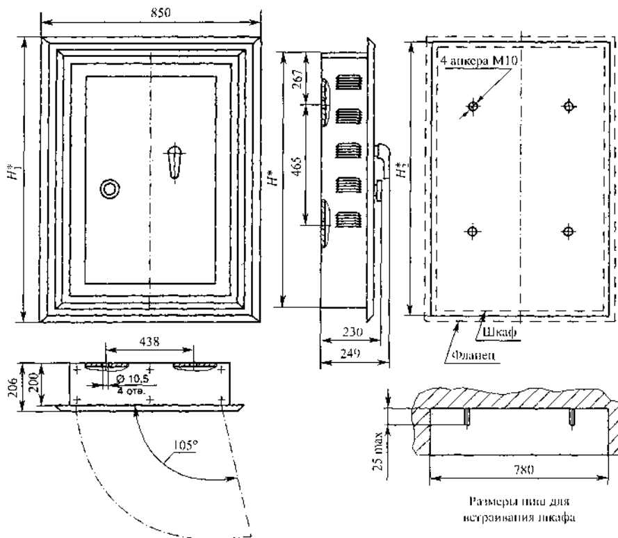
Рис. 7.3.4. Шкафы ПР 8804 углопенного исполнения
