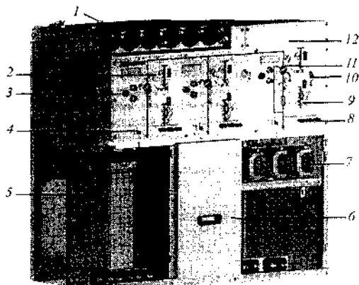
Рис. 6.4.2. Устройство моноблока «Ладога»: 1 — проушины для транспортировки; 2 — гнездо ручного оперирования заземляющим разъединителем; 3 — кнопки включения-отключения выключателя нагрузки (по отдельному заказу); 4 — рычаг блокировки двери отсека кабельных присоединений; 5 — отсек кабельных присоединений; 6 — низковольтный отсек; 7 — механический индикатор положения главных контактов; 8 — отключение выключателя защиты трансформатора; 9 — гнездо ручного оперирования выключателем; 10 — указатели наличия напряжения; 11 — держатели предохранителей; 12 — съемная дверь в кабельный отсек
