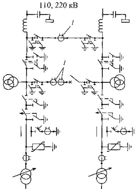
Рис. 3.4.13. Схема «мостик с выключателем в перемычке и отделителями в цепях трансформаторов»: 1 — трансформаторы тока, установка которых должна быть обоснована (индекс схемы — 5 по [26])
