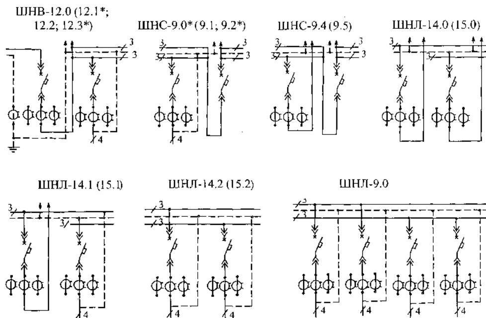
Рис. 4.3.12. Схемы соединений шкафов РУНН КТПП 2500 кВ·А производства Самарского завода «Электроцит»
