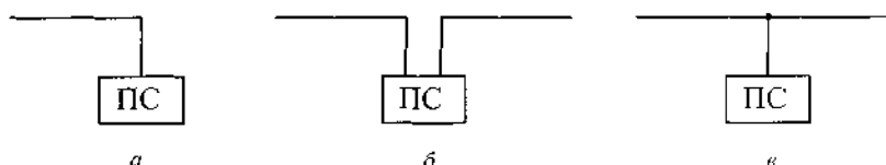
Рис. 3.1.1. Схемы присоединения подстанций к питающей линии а — тупиковая, б — проходная, в — ответвительная
