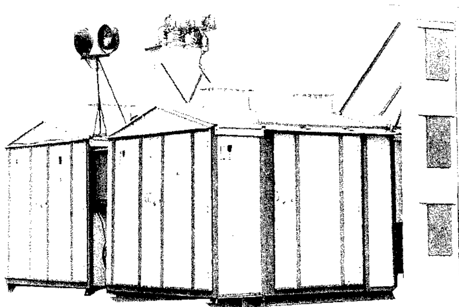
Рис. 4.3.15. Общий вид КТПГ производства ОАО «Самарский завод «Электроштит»
