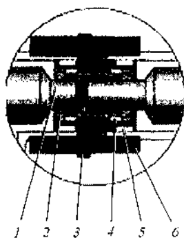
Рис. 6.2.15. Сборные шины КРУ/ТЕЛ: 1 — отрезки сборных шин; 2 — контакты цангового типа; 3 — изоляционная втулка; 4 — разрезные пружины; 5 — резиновые уплотнения; 6 — гайка из полимерного материала
