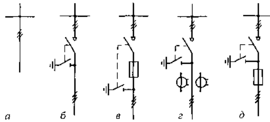
Рис. 4.3.5. Однолинейные схемы главных цепей УВН КТП 630 и КТП 1000 Чирчикского трансформаторного завода: а — ВВ-1; б — ШВВ-2-1; в — ШВВ-2-2; г — ШВВ-2-3; д — ШВВ-3
