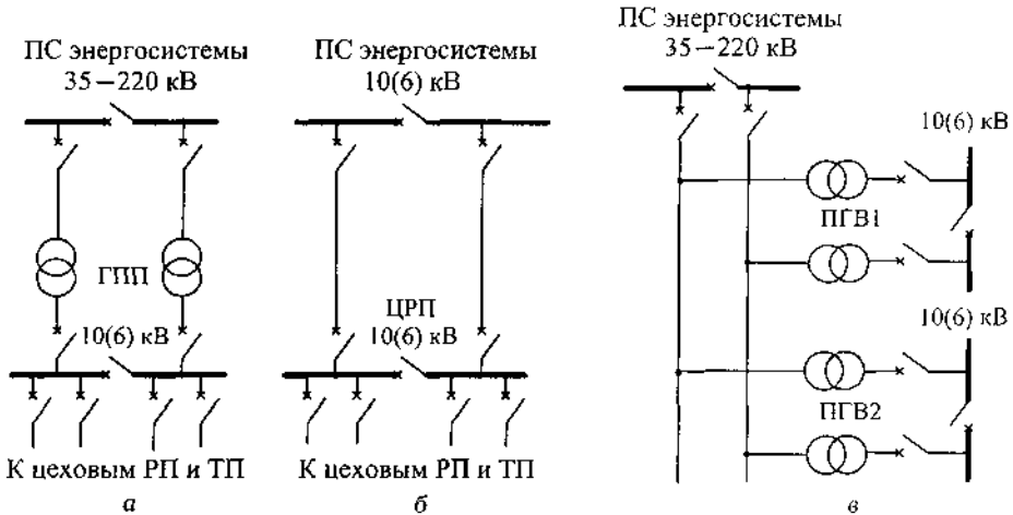
Рис. 1.6.5. Схемы внешнего электроснабжения предприятий средней мощности с приемным пунктом электроэнергии: а — ГПП; б — ЦРП; в — ПГВ.
