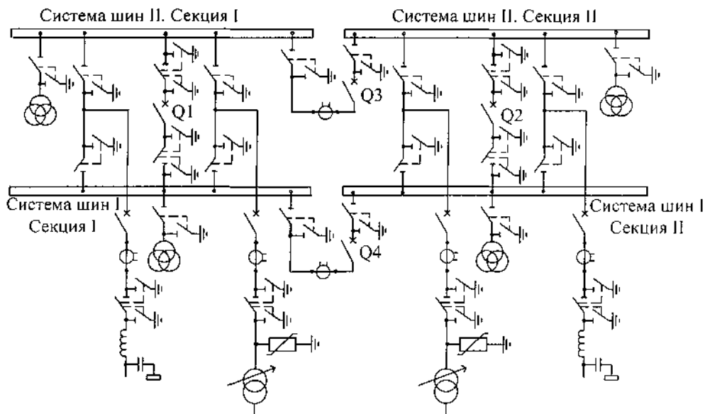
Рис. 3.4.8. Схема с двумя секционированными системами шин с двумя шинносоединительными ( Q_1 , Q_2 ) и двумя секционными ( Q_3 , Q_4 ) выключателями
