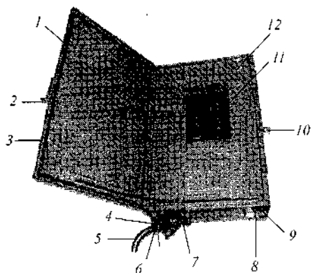
Рис. 6.5.22. Шкаф управления PBA/TEL: 1 — внешняя дверца; 2 — отверстие для навесного замка; 3 — резиновый уплотнитель; 4 — заземление; 5 — соединительный кабель; 6 — отверстие для кабеля дискретных входов (выходов); 7 — кабель питания; 8 — дренажный фильтр; 9 — отверстие для кабеля SCADA; 10 — отверстие для навесного замка; 11 — панель управления; 12 — внутренняя дверца
