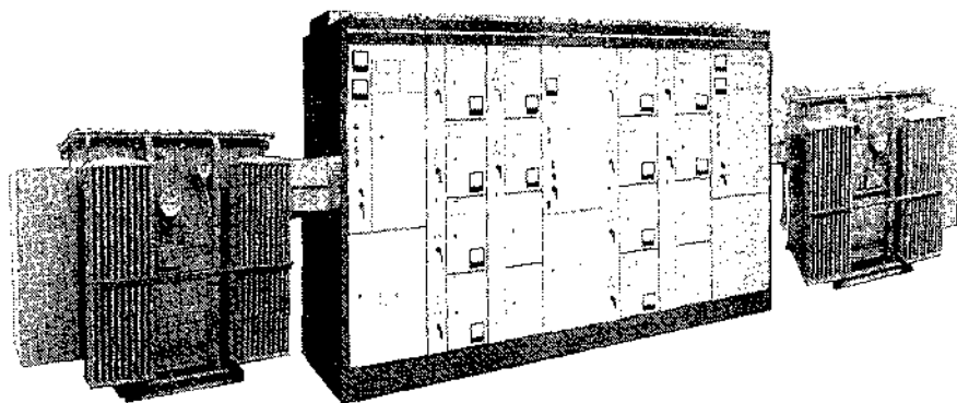
Рис. 4.3.13. Общий вид КТПП производства Самарского завода «Электроцит»
