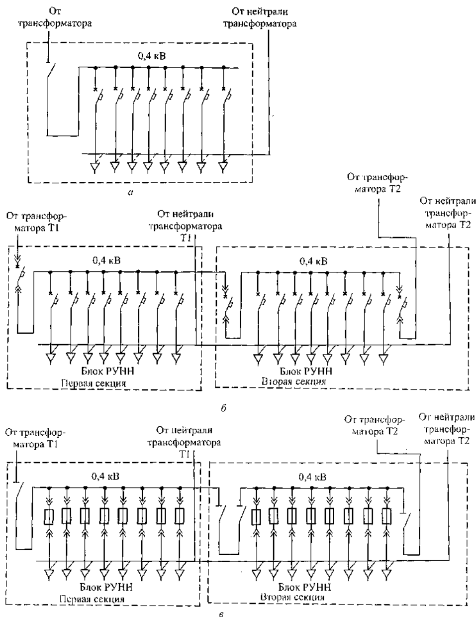
Рис. 4.3.21. Схемы РУНН КТПГ производства Самарского завода «Электрощит» (для вариантов 1, 6, 8 по табл. 4.3.17)
