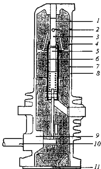
Рис. 6.6.7. Полос выключателя: 1 — корпус; 2 — изолирующее сопло; 3 — неподвижный дугогасительный контакт; 4 — главный подвижный контакт; 5 — подвижный дугогасительный контакт; 6 — подвижный поршень; 7 — камера сжатия; 8 — клапаны; 9 — система уплотнения; 10 — вал привода; 11 — нижняя крышка
