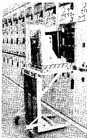
Рис. 6.3.23. Телжка-подъемник для перемещения выдвижных элементов
