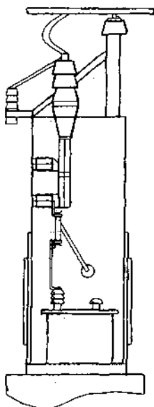
Рис. 6.5.2. Отдельно стоящий шкаф с ТСН по схеме 15 или 16 (УХЛ1)
