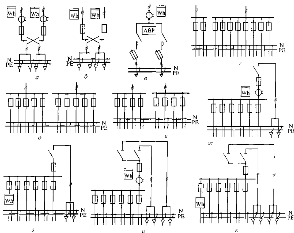
Рис. 7.4.1. Принципиальные схемы ВРУ-3: а, б, в — вводные; г, д, е — распределительные; ж, з, к, и — вводно-распределительные
