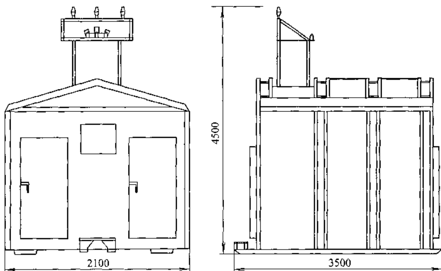
Рис. 4.3.30. Общий вид и габаритные размеры КТПК типа «киоск» производства «Самарского завода «Электрошит»
