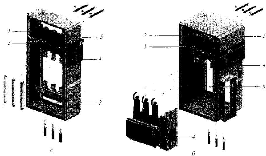
Рис. 6.6.2. Конструкция ячейки: a — с выключателем нагрузки и плавким предохранителем; б — с выключателем; 1 — отсек трехпозиционного разъединителя (выключателя нагрузки) и заземляющего разъединителя в одном корпусе; 2 — отсек сборных шин; 3 — кабельный отсек и отсек выключателя; 4 — отсек привода; 5 — отсек релейной защиты и цепей вторичной коммутации
