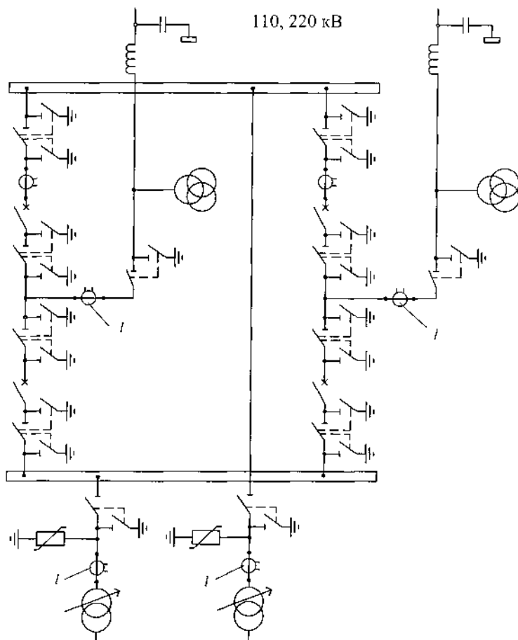
Рис. 3.4.17. Схема четырехугольника: 1 — трансформаторы тока, установка которых должна быть обоснована (индекс схемы — 7 по [26])
