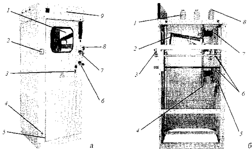
Рис. 6.2.1. Камера КСО-366М фирмы ALSTOM: а — общий вид (1 — смотровое окно; 2 — выключатель освещения (внутри ячейки); 3 — замок (блокировка, не позволяющая отпирать замок при включенном выключателе нагрузки); 4 — заземление; 5 — степень защиты IP20; 6 — поворотный повышенной безопасности привод заземлителя (пружинный); 7 — поворотный повышенной безопасности привод выключателя нагрузки (пружинный); 8 — поворотная механическая блокировка (замок Генодмана); 9 — поворотная панель клеммника вторичной коммутации); б — вид сбоку (1 — опорные изоляторы; 2 — направляющие инвентарной изолирующей перегородки; 3 — оперативная механическая блокировка (замок Генодмана); 4 — подключение кабеля (высота > 500 мм), число до 2 (алюминиевые жилы 180 мм 2 ); 5 — сборные шины; 6 — выключатель нагрузки ВН-10 (номинальный ток электродинамической стойкости 51 кА, ток термической стойкости 20 кА, пружинный привод); 7 — поворотные повышенной безопасности приводы выключателя нагрузки и заземлителей; 8 — заземлитель ЗР-10 (номинальный ток электродинамической стойкости 51 кА, термической стойкости 20 кА, пружинный привод)
