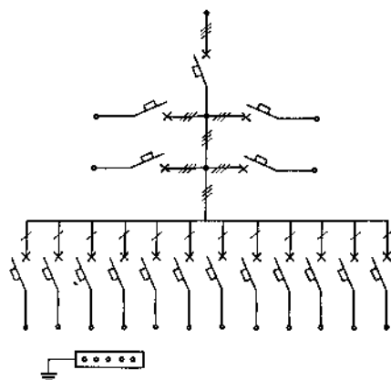
Схемы 217, 219, 240, 241 (число однополюсных автоматов – до 48)
