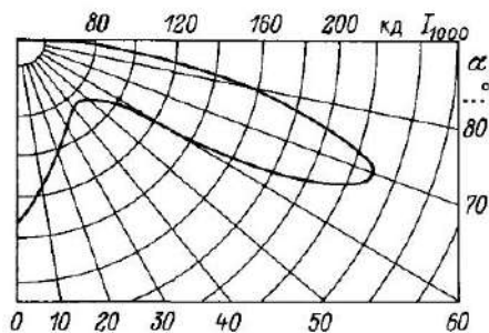
Рис 9 21 КСС светильников типа СЗПР-250МН-С
