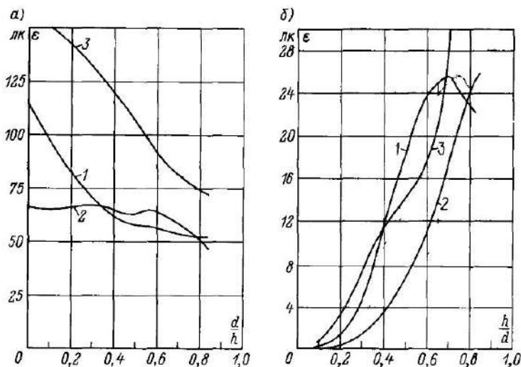
Рис 9.32 Кривые относительной освещенности светильников a - \epsilon = f(d/h) при d < h , b - \epsilon = f(h/d) при d > h 1 — СЗПР 250МН С, 2 — РТУ01 250/С53 02 У1, 3 — НКУ01 ( \beta=0 )
