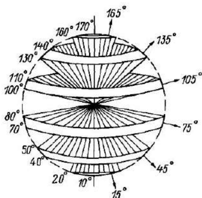
Рис 26 Зональные телесные углы (для десятиградусных зон)
