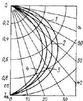
Рис 82 Тиловые кривые силы света светильников
