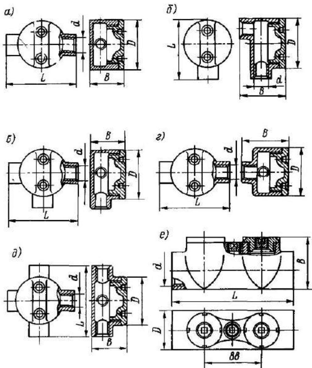
Рис. 14.7 Чугунные взрывозащищенные коробки серии В. а — проходные прямые типа КПП, б — проходные через дно (КПД), в — тройниковые осветительные (КТО); г — тройниковые с ответвлением через дно (КТД), д — крестовые ответвительные (ККО); е — проходные (КПЛ)
