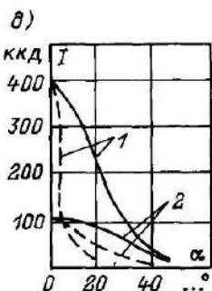
Рис 938 КСС прожекторов а — типа ПКН-1000Б (1) и ПКН-1500Б (2) в горизонтальной (—) и вертикальной (---) плоскости; б — типа ПСМ-40А-1 с лампами Г220-500, в — типа ПГП-М-3500 (1), ПГП-М-2000 (2); ПГП-М-1000 (3), г — типа ПГЦ-М-3500 в горизонтальной (—) и вертикальной (---) плоскости (1 — с зеркальным отражателем, 2 — с ячеистым отражателем); д — типа ПГЦ-М-2000; е — типа ПГЦ-М-1000
