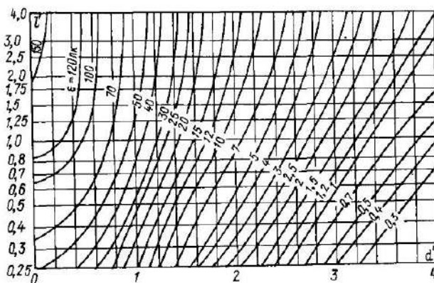
Рис 730 Линейные изолюксы для светильников с КСС типа Д-1
