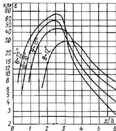
Рис 9 50 Приведенная освещенность от веера прожекторов ПСМ-50А-1 с лампами КГ220-1000
