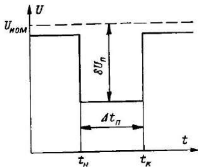
Рис 11.2. Провал напряжения
