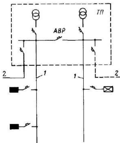
Рис 11.11. Схема питания осветительной сети при системе трансформатор — магистраль 1 — главные магистрали, 2 — линии, питающие внещевые нагрузки
