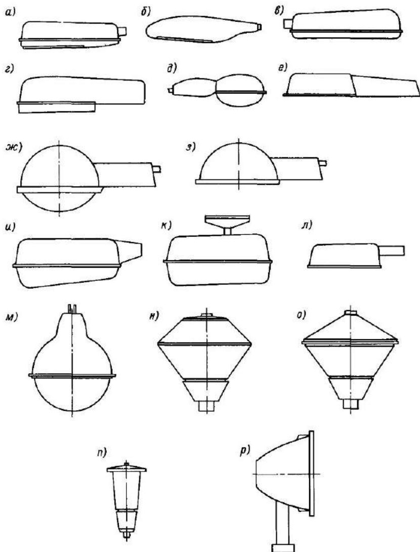
Рис 9.1. Внешний вид светильников типа: а — РКУ01-250-007-У1 и РКУ01-250-009-У1, б — РКУ01-250-011-У1, в — ЖКУ01-250-004-У1 и ЖКУ01-400-002-У1, г — ЖКУ02-400-003-УХЛ1 и ЖКУ02-400-004-УХЛ1, д — РКУ03, ГКУ03, ЖКУ03; е — РКУ06-125-001-У1; ж — РКУ07, ЖКУ07, модификация 001; з — РКУ07, ЖКУ07, модификация 002; и — ЖКУ08-150-001-УХЛ1, к — РСУ08-250-001-У1, л — НКУ01-200/Д23-02, м — СЗПР-250МН, н — РТУ01-250/С53-01-У1, о — РТУ01-250/С53-02-У1; п — РТУ02; р — ИСУ02-5000/К23-01-ХЛ1
