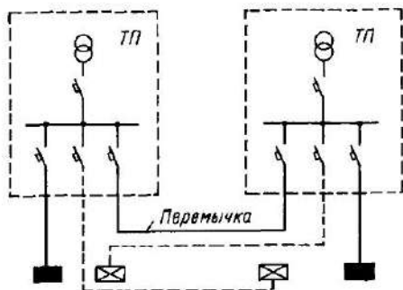
Рис. 11.8 Схема питания осветительной сети от двух однострансформаторных подстанций с перемычкой между ними на стороне низшего напряжения
