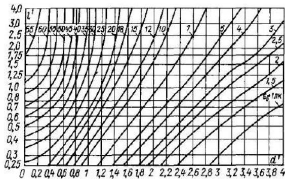
Рис 7.34 Линейные изолюксы условной горизонтальной освещенности E_0
