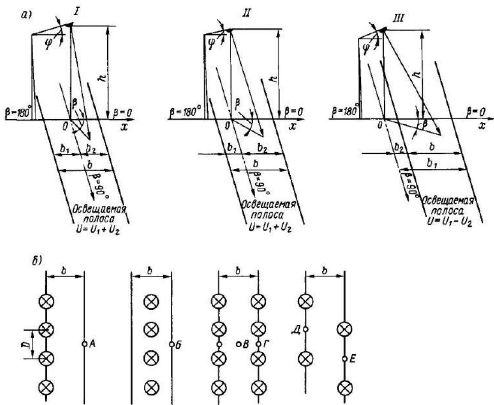
Рис 9.31 Расположение светильников относительно освещаемой поверхности а — к определению коэффициента использования, б — расположение точек минимальной освещенности (А, Б, В, Г, Д)
