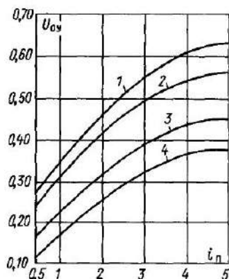
Рис. 6.1. Графики зависимости коэффициента использования ОУ от индекса помещения
