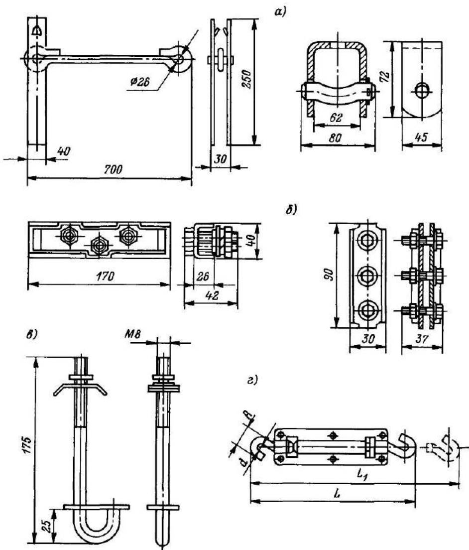
Рис 13 11 Изделия для крепления тросов а — анкеры К809 и К675, б — зажимы К676 и К296, в — серьга К1016, г — натяжная муфта
