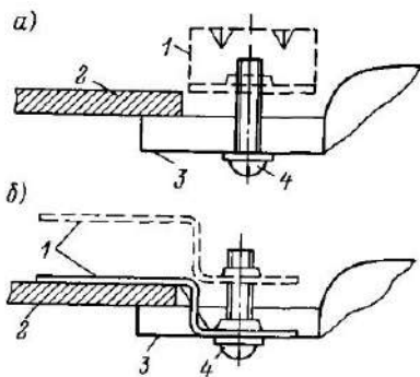
Рис 14 б Крепление встраиваемых светильников, обслуживаемых снизу, поворотными скобами а — при установке светильника, б — при его закреплении
