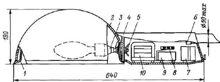
Рис П 8 Конструкция светильников типа РКУ07, ЖКУ07, модификация 002 1 — 10 — то же, что на рис П 7
