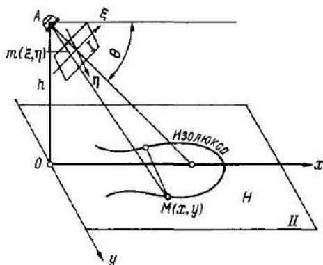
Рис 9.40 Построение изолукс
