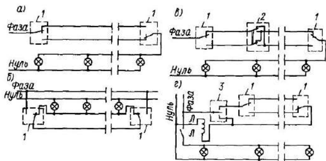
Рис 11.17 Коридорные схемы управления освещением а — из двух мест, б — из двух мест с транзитной фазой, в — из трех мест (а при увеличении числа выключателей 2 — из любого числа мест), г — с помощью пускателей, реле или контакторов (при управлении их катушками применяются схемы а , б , в )
