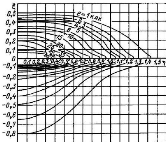
Рис 9.47 Изолюксы на условной плоскости для светильника прожекторного типа ИСУ01-2000
