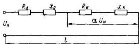
Рис 12.14 Схема замещения линии управления освещением с индуктивностью
