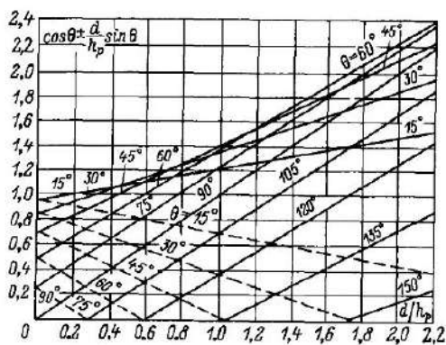
Рис 7.49 Номограмма для определения \psi (d/h_p)
