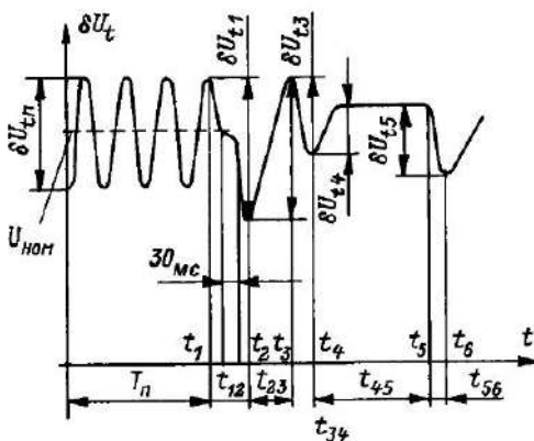
Рис 11.1. Колебания напряжения \delta U_{1n} — размах периодических колебаний (семь «размахов» за время T_n ), \delta U_n \div \delta U_{15} — размах неперiodических колебаний
