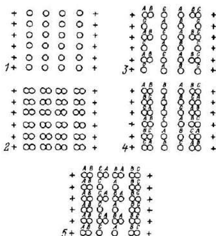
Рис 3.3 Схемы четырехрядного размещения светильников с разрядными лампами высокого давления (ДРЛ, МГЛ и ДНаТ) «+» — колонна, O — светильник, А, В, С — фазы электрической сети
