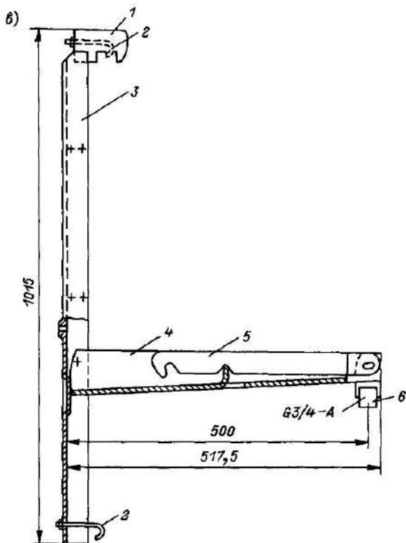
Рис 13.16 Поворотные кронштейны а — КПК, б — КЛТ, в — КЛШ
