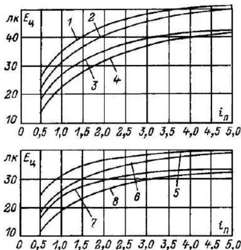
Рис 8.4 График зависимости минимальной цилиндрической освещенности от индекса помещения для светораспределения I_\alpha = I_0 \cos \alpha при удельном световом потоке F_\gamma = 100 \text{ лм/м}^2
