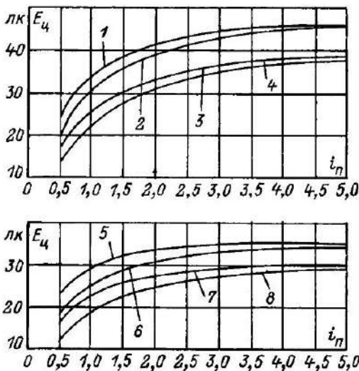
Рис 8.5 График зависимости минимальной цилиндрической освещенности от индекса помещения для светораспределения I_\alpha = I_0 \cos^2 \alpha при удельном световом потоке F_\gamma = 100 \text{ лм/м}^2
