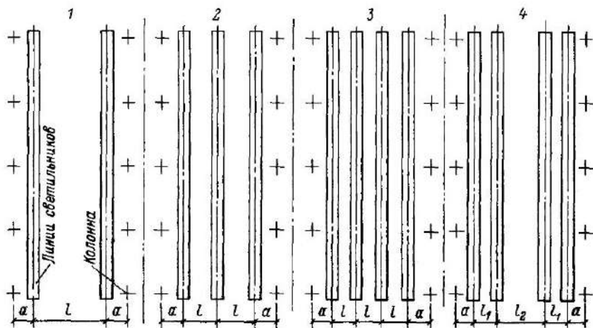
Рис 31 Схемы размещения линий светильников с люминесцентными лампами 1—3 — равномерное размещение линий по помещению, 4 — линии сдвинуты к стенам
