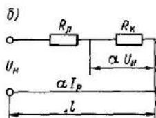
Рис 12.15 Схемы замещения линии управления постоянного тока
