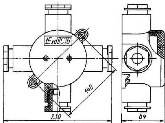
Рис 14 9 Коробка ответвительная взрывозащищенная КВП-25
