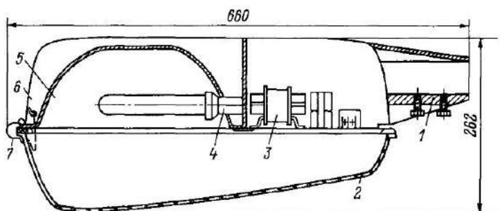
Рис. П 9. Конструкция светильников типа ЖКУ08-150-001-УХЛ1 1 — консоль, 2 — защитное стекло, 3 — ПРА, 4 — патрон, 5 — алюминиевый отражатель, 6 — корпус, 7 — защелки
