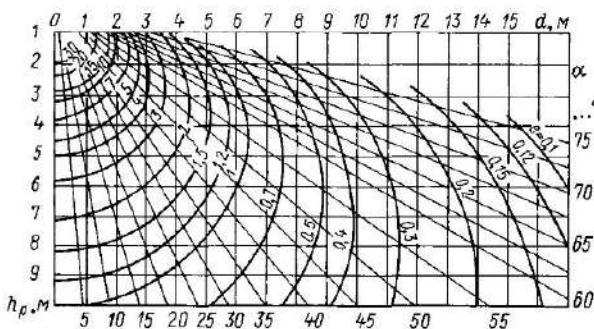
Рис 7 21 Пространственные изолуоксы горизонтальной освещенности (сила света светильника по всем направлениям 100 кд)
