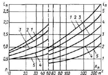
Рис. 8.3 Зависимость индекса помещения i_n от площади помещения при различной высоте его h_p
