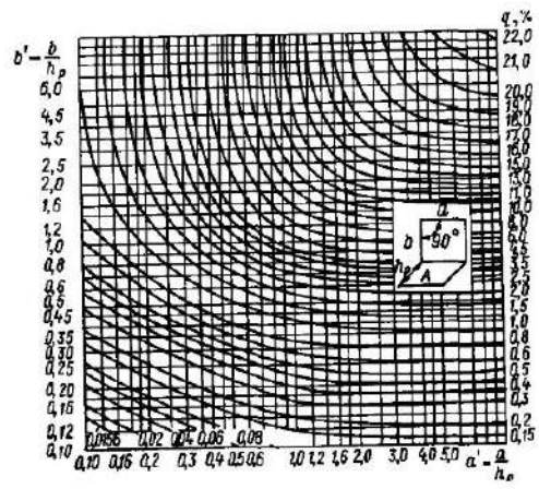
Рис. 7.33. Линейные изолюксы для светильников КСС типа Д
