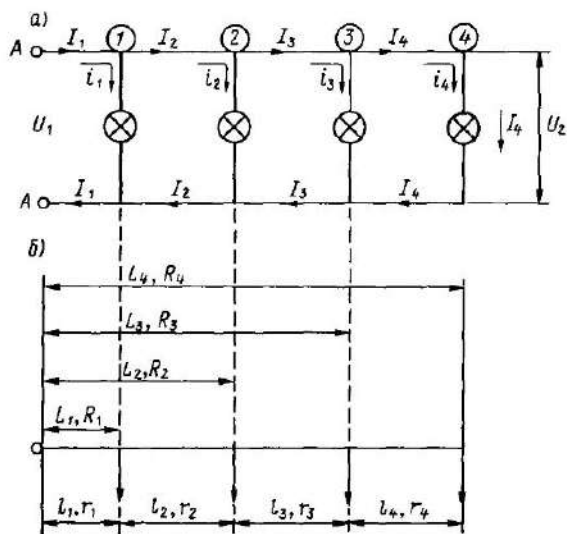
Рис 12.1 К определению потерь в двухпроводной линии i_1 - i_4 — нагрузочные токи, A , I_1 - I_4 — токи, проходящие по отдельным участкам линии, A , l_1 - l_4 — длины отдельных участков линии, m , r_1 - r_4 — сопротивление проводов отдельных участков линии, L_1 - L_4 , R_1 - R_4 — длины отрезков линии от источника питания до точки приложения нагрузки и их сопротивления
