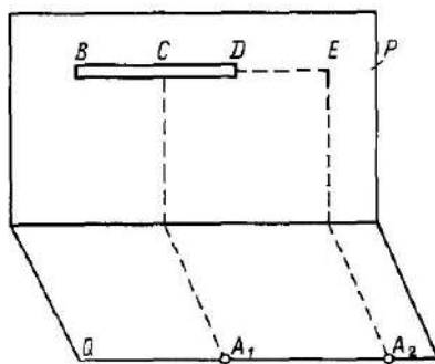
Рис 7.26 Освещенность точек, не лежащих против конца линии
