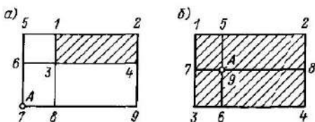
Рис 7.46 Схемы размещения светящих прямоугольников относительно расчетной точки
