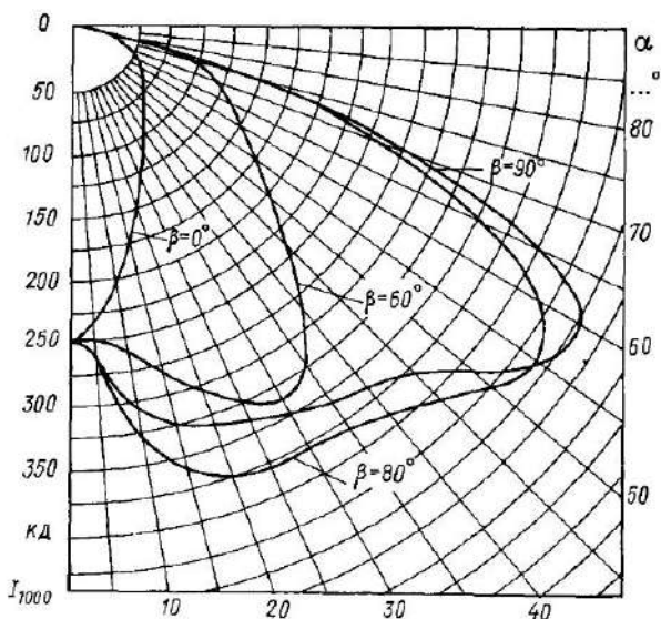
Рис 9.12 КСС светильников типа ГКУ03-250-001-У и ГКУ03-400-003 У
