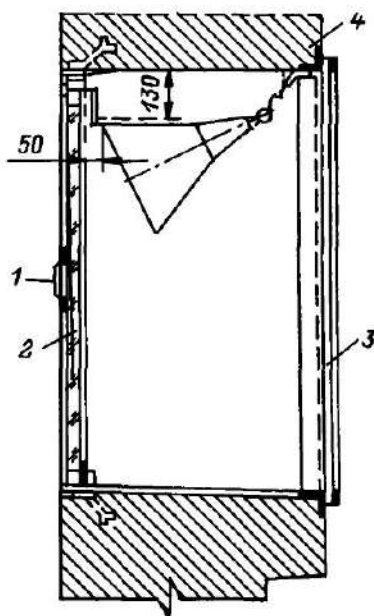
Рис 14.13. Освещение помещения светильником, установленным в стенной нише
