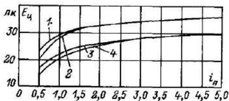
Рис 88 График усредненных значений отношения горизонтальной освещенности к цилиндрической зависимости от индекса помещения для светораспределения I_\alpha = I_0 \cos \alpha
