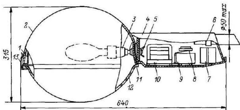
Рис П 7 Конструкция светильников серий РКУ07, ЖКУ07, модификация 001 1 — отражатель, 2 — корпус, 3 — патрон, 4 — корпус электротехнического отсека, 5 — штуцер, 6 — узел крепления, 7 — компенсирующие конденсаторы, 8 — зажимы, 9 — импульсное зажигающее устройство, 10 — ПРА, 11 — уплотнительное кольцо, 12 — защитное стекло; 13 — замки
