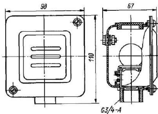
Рис 13 20 Коробка-амортизатор К937
