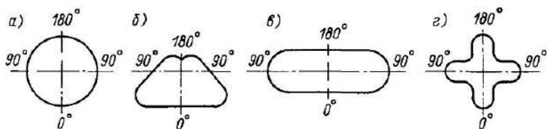
Рис 9.30 Характер изолукс на горизонтальной плоскости и отсчет угла \beta светильников наружного освещения а — симметричное светораспределение (С), б — боковое светораспределение (В), в — осевое светораспределение (I), г — для площадей (II)
