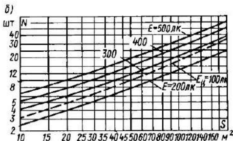
Рис 6.2 График для определения числа светильников типа ЛСП02 с лампами ЛБ40 при коэффициентах отражения \rho_n = 70\% , \rho_c = 50\% , \rho_p = 10\% а — h = 1,5 \div 2 \text{ м} , б — h = 2 \div 3 \text{ м}
