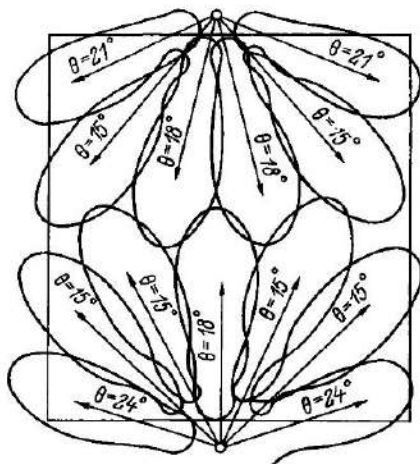
Рис 9.48 Пример компоновки изолюксы
