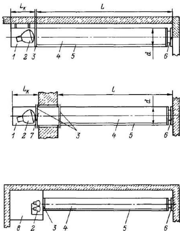
Рис 54 Комплексные осветительные устройства со шелевым световодом а — КОУ1, б — КОУ1А, в — КОУ1С 1 — камера, 2 — источник света, 3 — прозрачный иллюминатор, 4 — канал шелевого световода, 5 — оптическая щель, 6 — торцевой элемент, 7 — переходный элемент, 8 — строительная галерея
