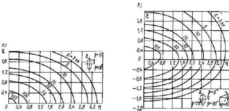
Рис. 9.33 Графики условных изолюкс. а — для светильников типа РСУ05 с лампами ДРЛ ( \Phi_0 = 1000 лм), б — для светильников типа РКУ01 с лампами ДРЛ ( \Phi_0 = 1000 лм, \varphi = 15^\circ )
