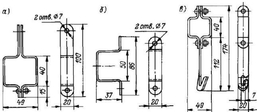
Рис 13.12 Конструкции для крепления осветительных шинопроводов ШОС2 и ШОС4 а — хомут К544, б — скоба К474, в — хомут с крюком К470
