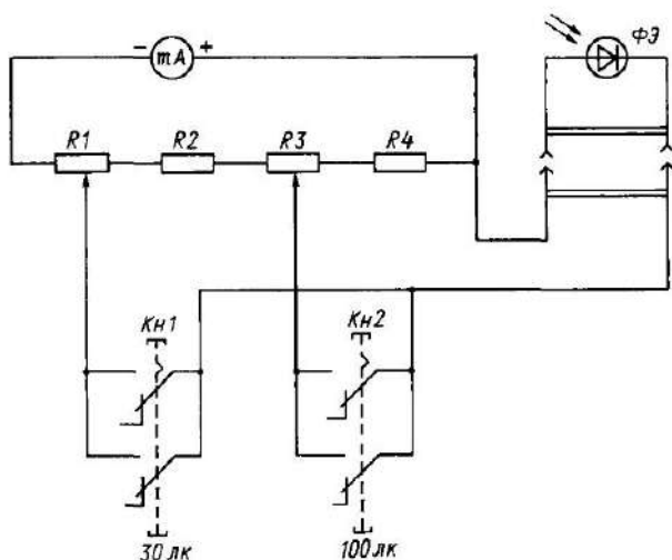
Рис 14 15 Принципиальная электрическая схема люкметра Ю116
