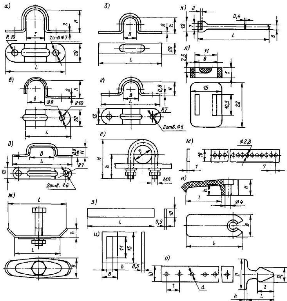
Рис. 13.10 Изделия для крепления кабелей, проводов и труб а — скобы К142 — К145, б — скобы К146п — К148п, в — скобы К252 — К254, г — скобы К729 — К731, д — скобы К732 — К740, е — хомутки ХТС, ж — накладки НТ, з — полоски К404, К405, и — пряжка К407, к — полоски пряжки К395 — К398, л — закладная пряжка Л165, м — лента К226, н — скоба К641, К642, о — монтажная лента ЛМ и замок для нее
