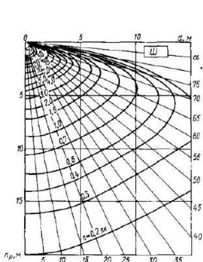
Рис 7.8 Пространственные изолюксы условной горизонтальной освещенности от светильников с КСС типа Ш
