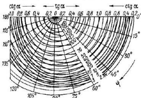
Рис 7.23 Изолюксы относительной освещенности (прожектор ПЗР-400 с лампой ДРЛ)
