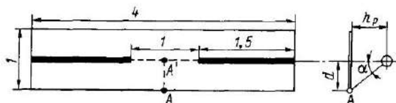
Рис 7.40 К примеру 7.7 (размеры — в метрах)
