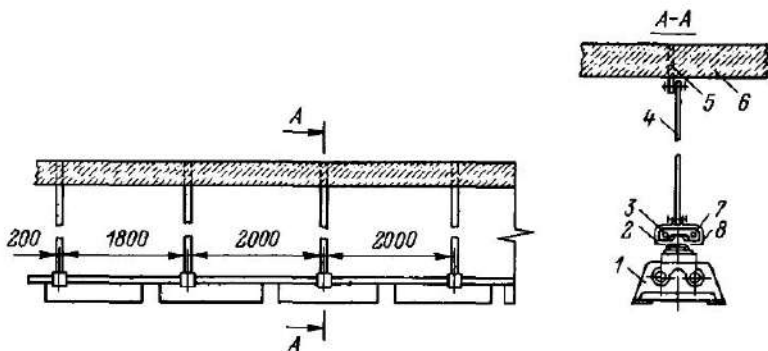
Рис 14.3 Установка светильников на коробах КЛ-1
