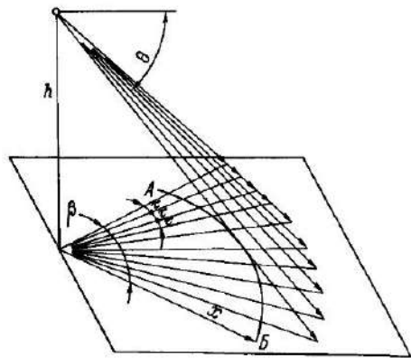
Рис 9.49 Пучок прожекторов
