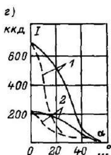
Рис 938 КСС прожекторов а — типа ПКН-1000Б (1) и ПКН-1500Б (2) в горизонтальной (—) и вертикальной (---) плоскости; б — типа ПСМ-40А-1 с лампами Г220-500, в — типа ПГП-М-3500 (1), ПГП-М-2000 (2); ПГП-М-1000 (3), г — типа ПГЦ-М-3500 в горизонтальной (—) и вертикальной (---) плоскости (1 — с зеркальным отражателем, 2 — с ячеистым отражателем); д — типа ПГЦ-М-2000; е — типа ПГЦ-М-1000
