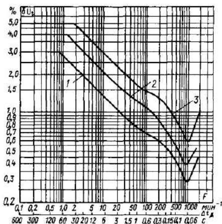
Рис 11.5. Допустимый размах изменений напряжения ( \delta U_n , %) в зависимости от частоты или интервала времени ( \Delta t_d , с) между изменениями напряжения
