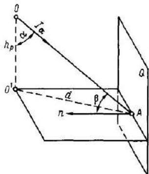
Рис 7.48 К расчету освещенности вертикальной плоскости
