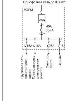
Схема «Минимал»
