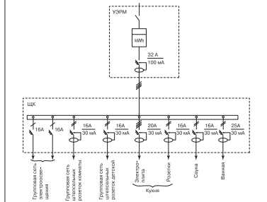
Схема «Экстра»
