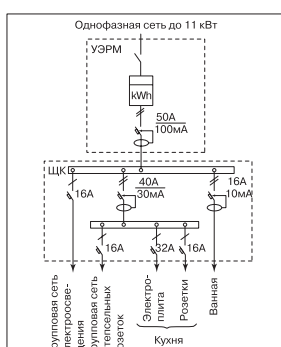
Схема «Оптималь»
