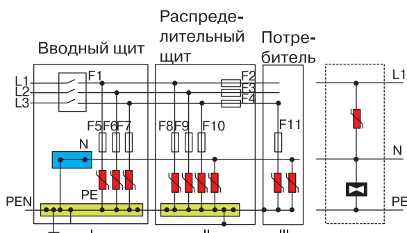
Установка УЗИП в сети TN-C-S 220/380 В.
