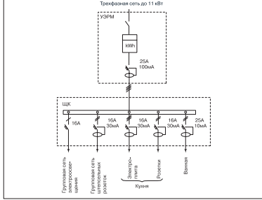
Схема «Трико»
