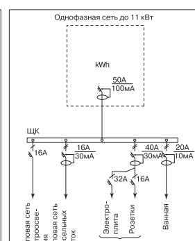
Схема «Комфорт»
