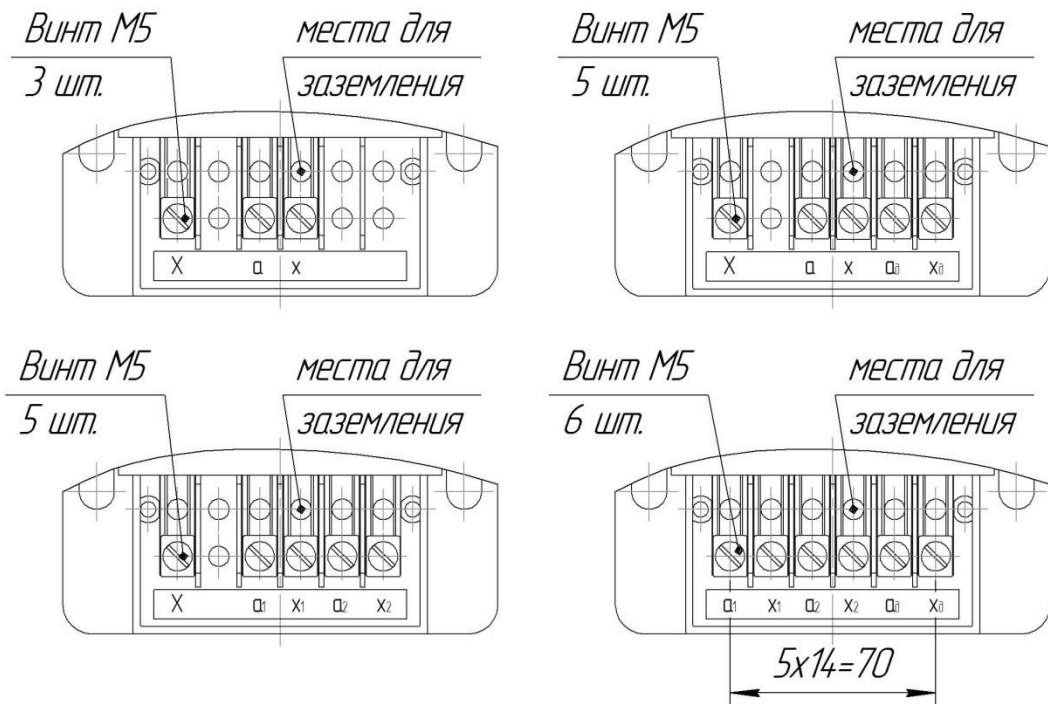
Рисунок 7 - Расположение вторичных выводов трансформаторов ЗНОЛ-СЭЩ-6(10)
