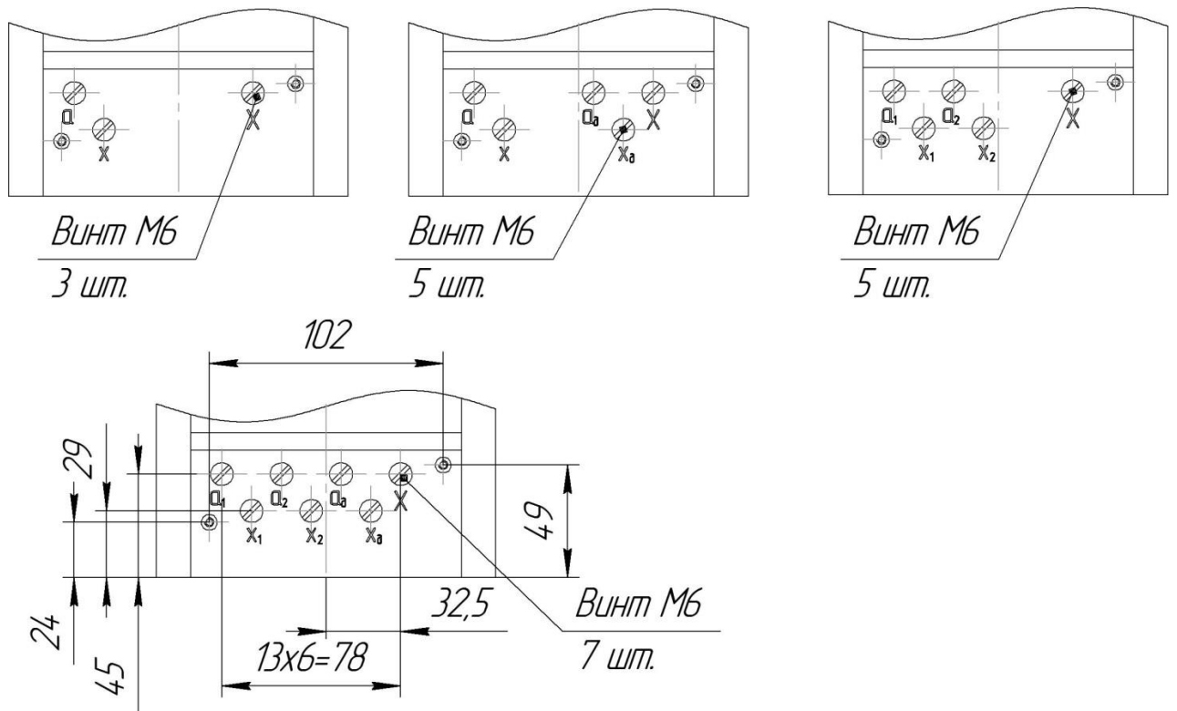
Рисунок 9 - Расположение вторичных выводов трансформаторов ЗНОЛ-СЭЩ-6(10)-20
