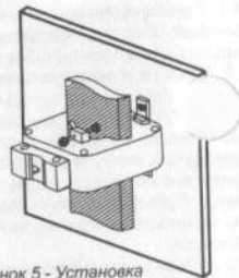
Рисунок 5 - Установка трансформаторов модификации ТТЭ-85, ТТЭ-100, ТТЭ-125 на шине при помощи крепежной пластины и винтов.
