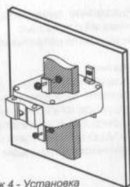
Рисунок 4 - Установка трансформаторов модификации ТТЭ-30, ТТЭ-40, ТТЭ-60 на шине при помощи крепежной пластины и винтов.
