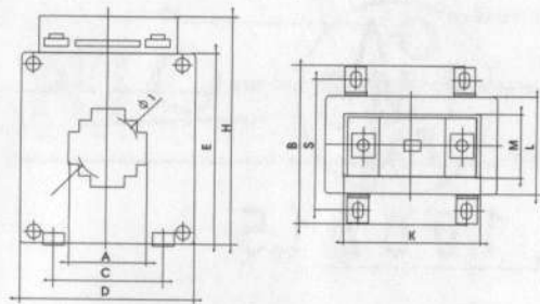
Рисунок 2 — Габаритные и установочные размеры модификации ТТЭ-30, ТТЭ-60, ТТЭ-100, ТТЭ-125
