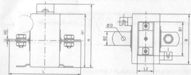
Рисунок 1 — Габаритные и установочные размеры модификации ТТЭ-А
